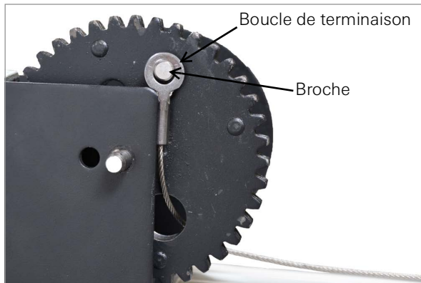
ILLUSTRATION 45: Retirez la boucle de terminaison
