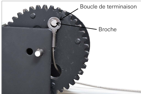
ILLUSTRATION 41: Retirez la boucle de terminaison
