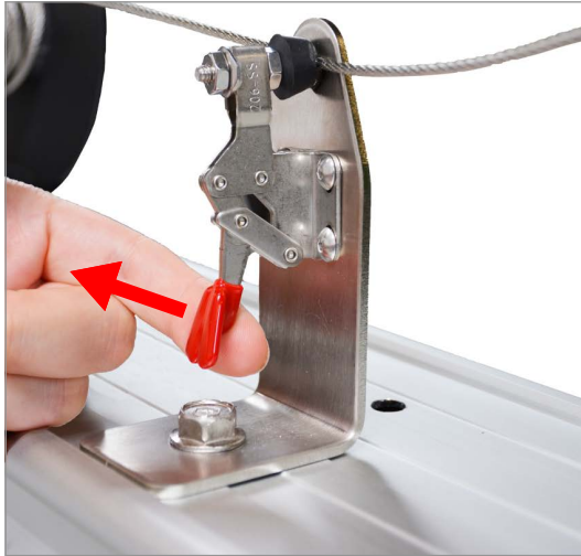
ILLUSTRATION 39: Relâchez la pince centrale
