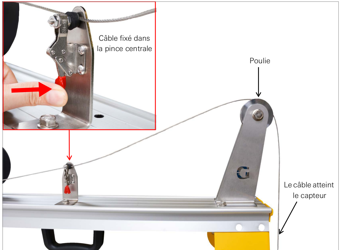
ILLUSTRATION 37: Câble de support aligné sur la poulie et fixé dans la pince centrale
