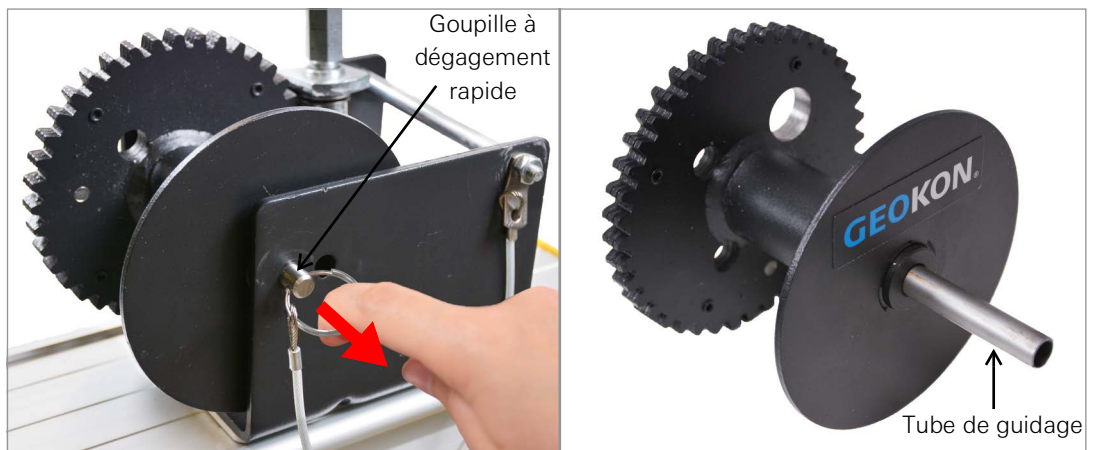
ILLUSTRATION 43: Retirez l'enrouleur vide et le tube de guidage
