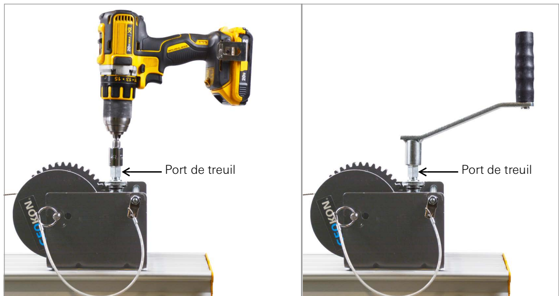
ILLUSTRATION 48: Perceuse (à gauche) ou poignée manuelle (à droite) installée sur le port de treuil
