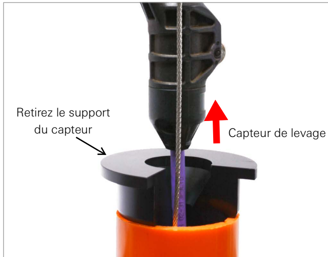
ILLUSTRATION 40: Capteur soulevé du support de capteur
