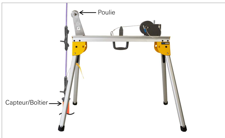
ILLUSTRATION 35: Cadre modèle 6140-HOIST
