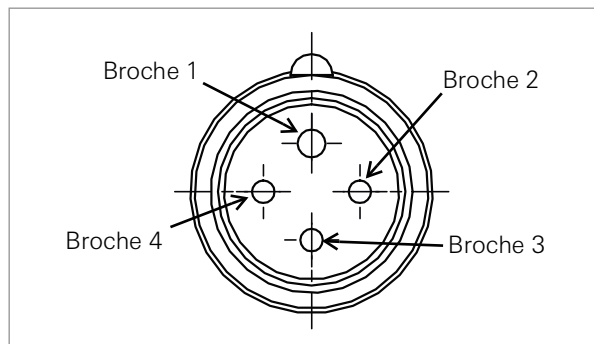
ILLUSTRATION 16: Connecteur femelle étanche
