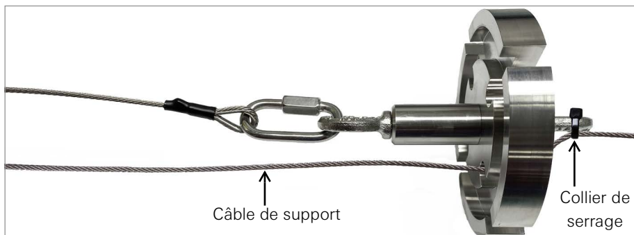
ILLUSTRATION 46: Fixez l'extrémité de terminaison au support de suspension
