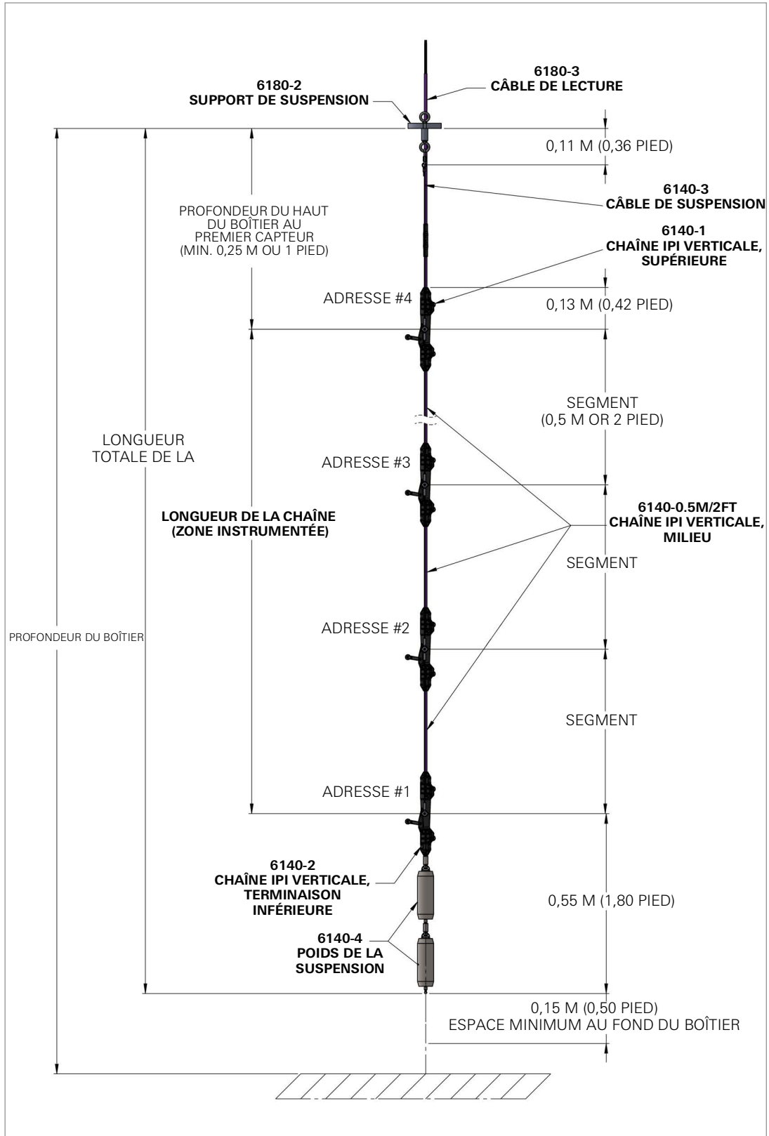
ILLUSTRATION 27: Diagramme d'assemblage standard (Chaîne de plus de 50 capteurs illustrée)
