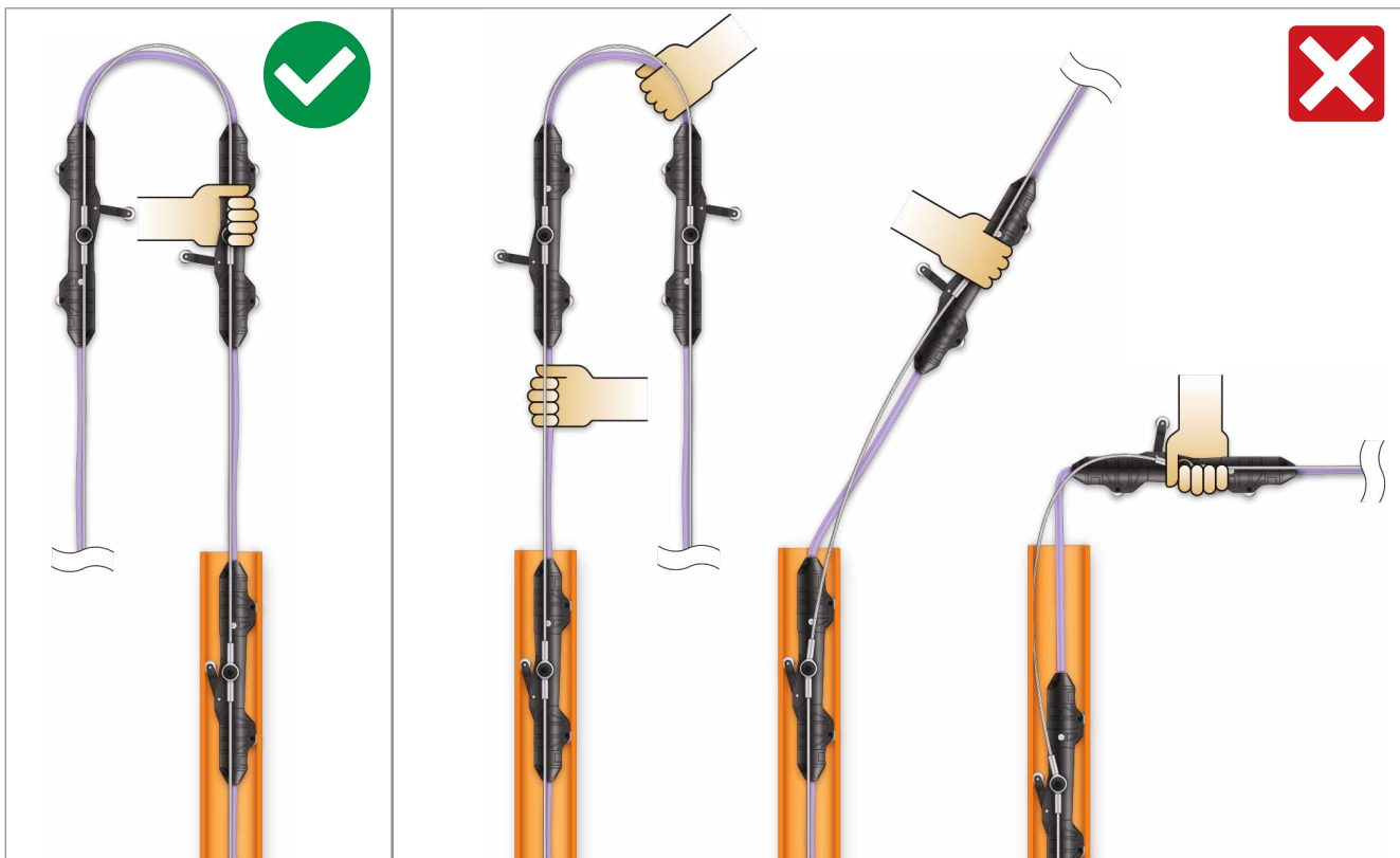
FIGURE 8: Orientation du capteur
