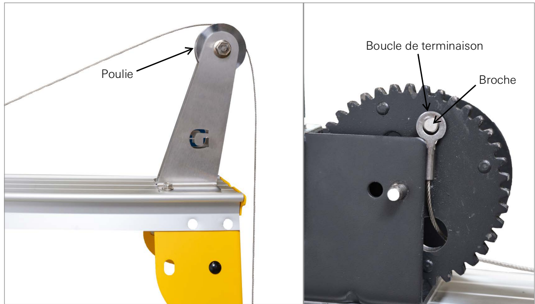
ILLUSTRATION 49: Câble de support sur poulie (à gauche) et boucle de terminaison installée sur enrouleur vide (à droite)
