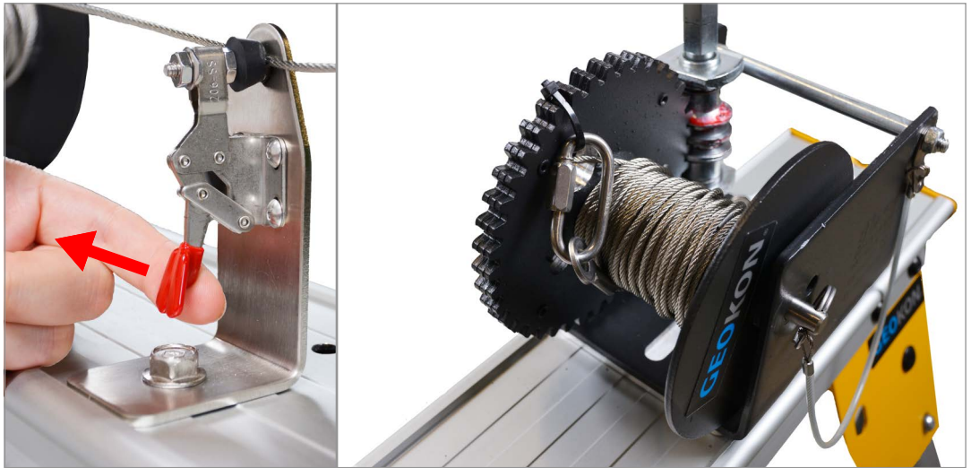
ILLUSTRATION 52: Relâchez la pince centrale (à gauche) et fixez le câble de support à l'enrouleur (à droite)
