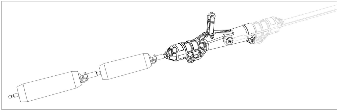
ILLUSTRATION 20: Chaîne verticale IPI inférieure modèle 6140-2, avec (2) poids de suspension modèle 6140-4 fixés
