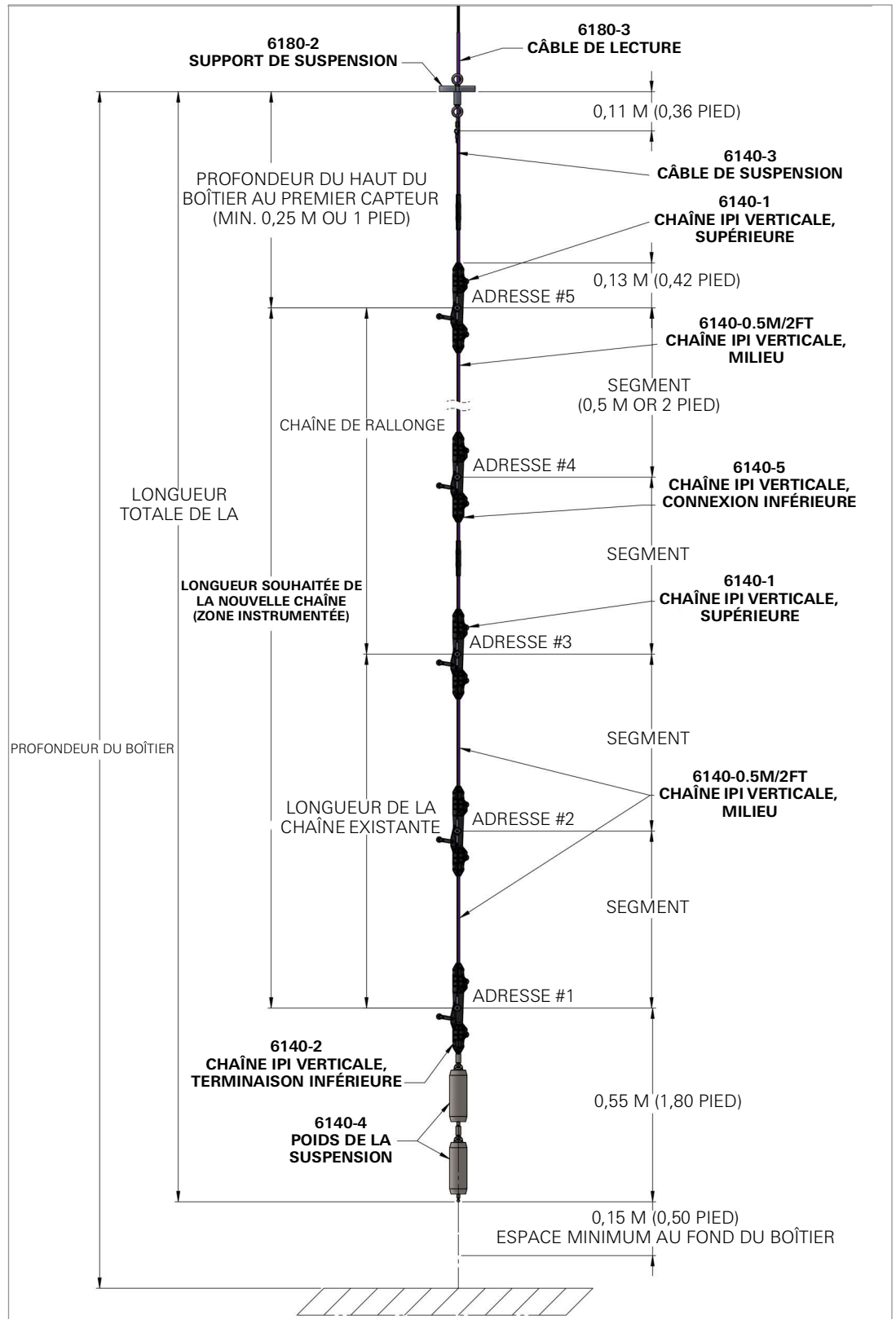
ILLUSTRATION 28: Diagramme d'assemblage de rallonge (Chaîne de plus de 50 capteurs illustrée)
