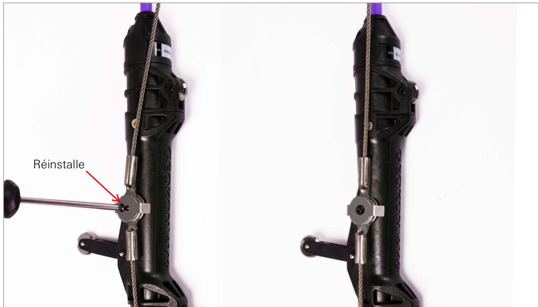
ILLUSTRATION 12: Œillets de câbles d'aéronef sécurisés, connexion de câbles d'aéronef terminée
