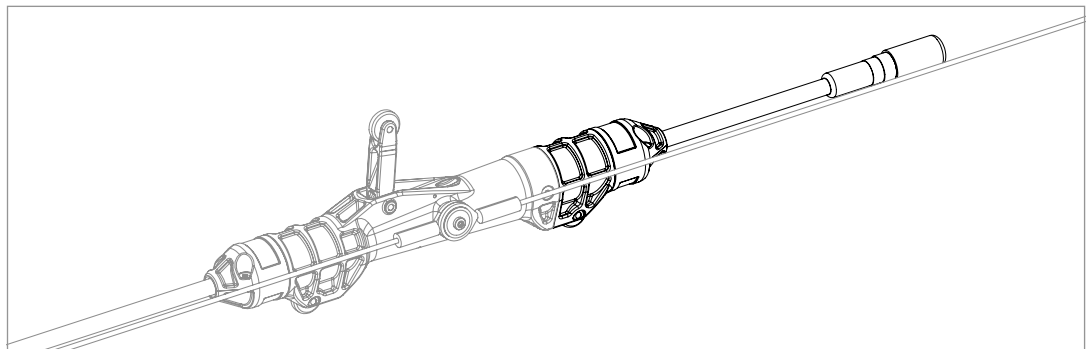
ILLUSTRATION 18: Chaîne verticale IPI supérieure modèle 6140-1, avec connecteur de câble de lecture
