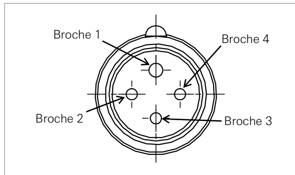
ILLUSTRATION 15: Connecteur mâle étanche
