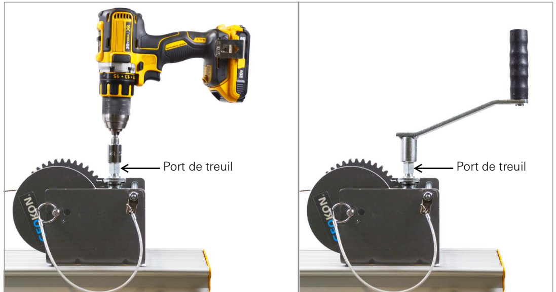
ILLUSTRATION 36: Perceuse (à gauche) ou poignée manuelle (à droite) installée sur le port du treuil
