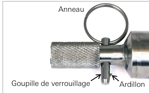
ILLUSTRATION 2: Détails de la goupille de verrouillage
