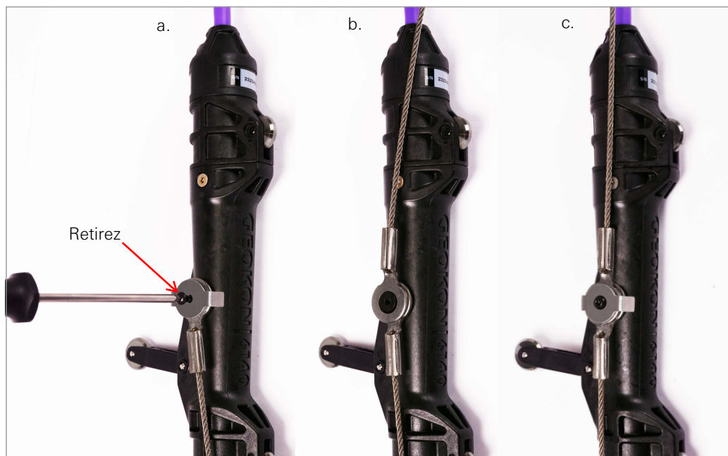
ILLUSTRATION 7: Connexion du câble d'aéronef
